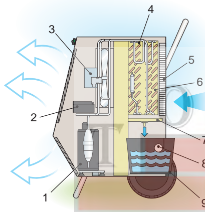
Fig. 1. Schema funzionale: 1. Compressore ermetico; 2. Apparecchiatura di controllo; 3. Ventilatore elicoidale; 4. Condensatore; 5. Filtro dell'aria; 6. Evaporatore; 7. Raccordo di scarico; 8. Galleggiante; 9. Serbatoio dell'acqua (Eccetto DH 80).
